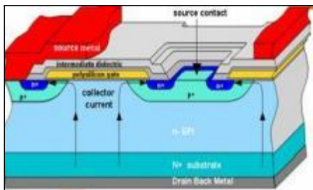
特高压平面MOSFET结构
